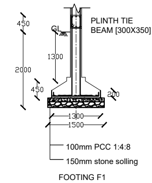
FOOTING F1
