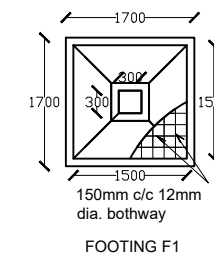
FOOTING F1
