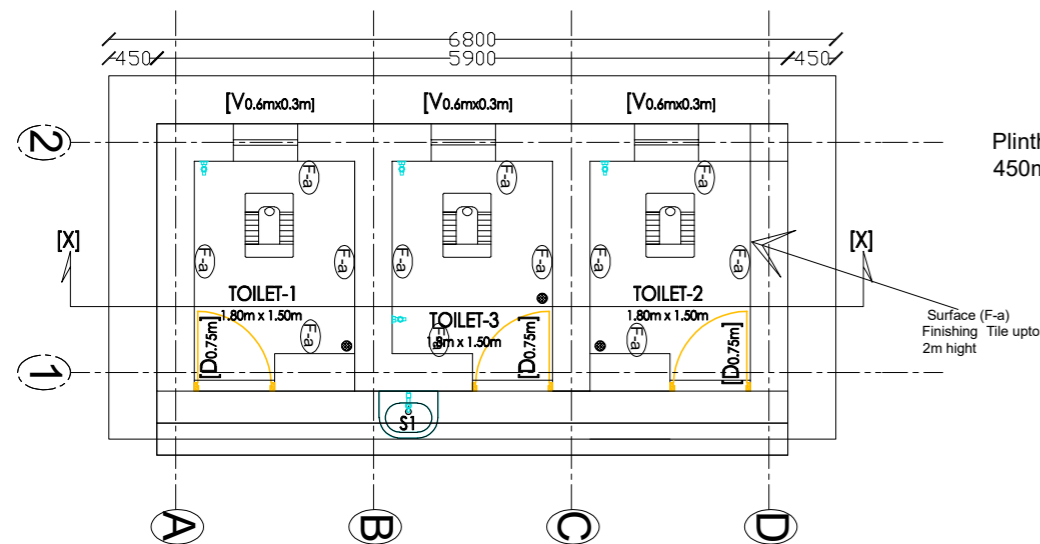
Toilet Plan
