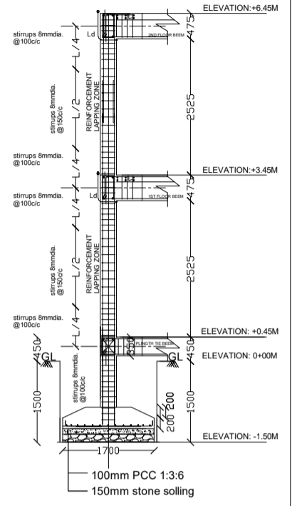
FOOTING & COLUMN F1 Type
